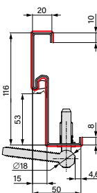
ACÉL SAROK AJTÓTOK
