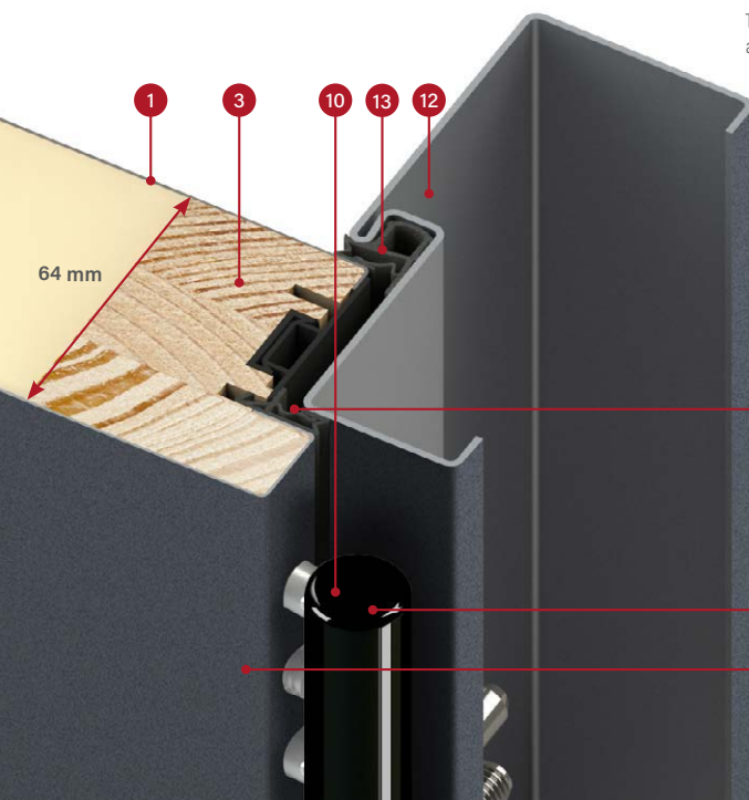
THERMO 64 ajtószárny acél ajtótokjának keresztmetszete
