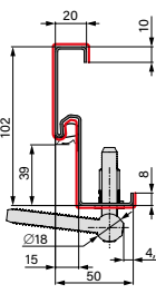
ACÉL SAROK AJTÓTOK
