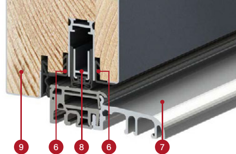
THERMO 64 ajtószárny keresztmetszete takaró tömítéssel és anélkül, alumínium küszöb
