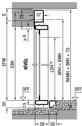
Függőleges metszet
