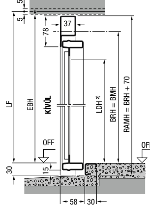
Függőleges metszet
