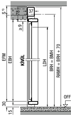
Függőleges metszet
