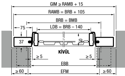
Vízszintes metszet
