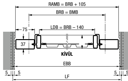
Vízszintes metszet
