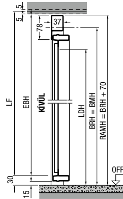
Függőleges metszet
